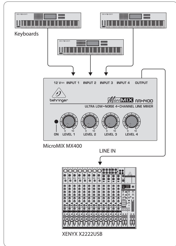
Example: MX400 wiring
